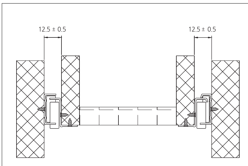
철 레일 장착 도면 | Drawing
