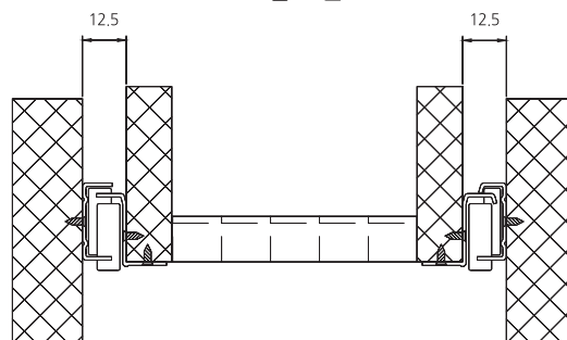
조립도면
