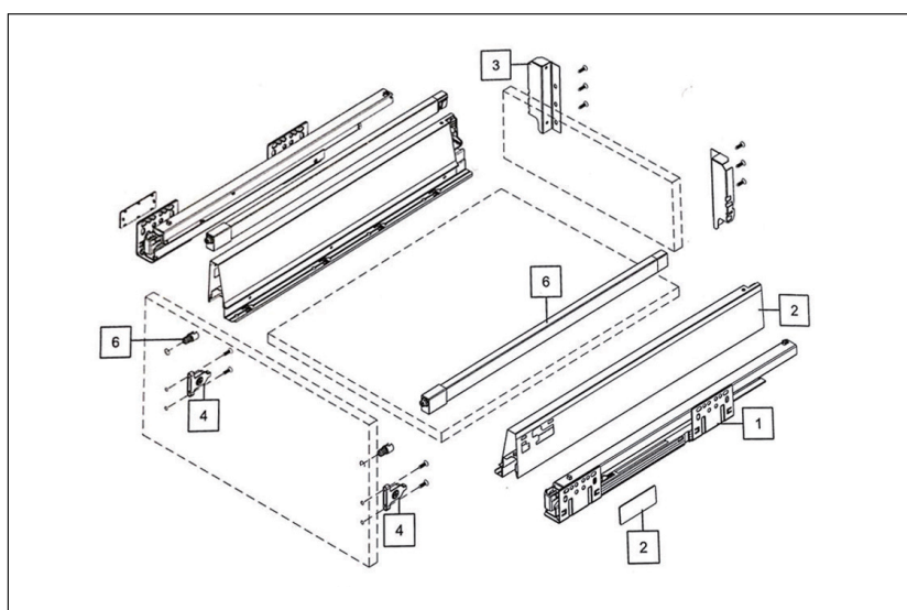
제품 도면 | Drawing
