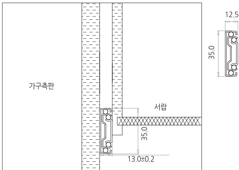
제품도면 | Drawing
